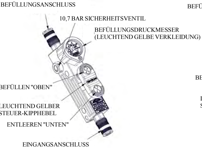
Abbildung 1-4. 10.34 bar ALB-Einzelsteuerung G2
