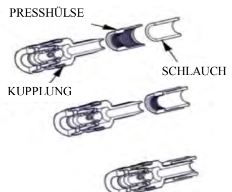
Abbildung 3-2 Austausch der Luftschlauch-Schnellkupplung
